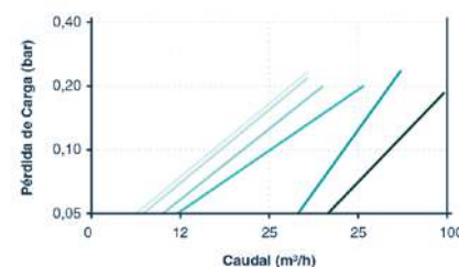
Pérdida de Carga Filtro Anillas
